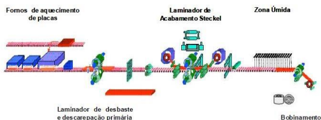
Figura 1: Redução e refino dos aços GO e GNO.
